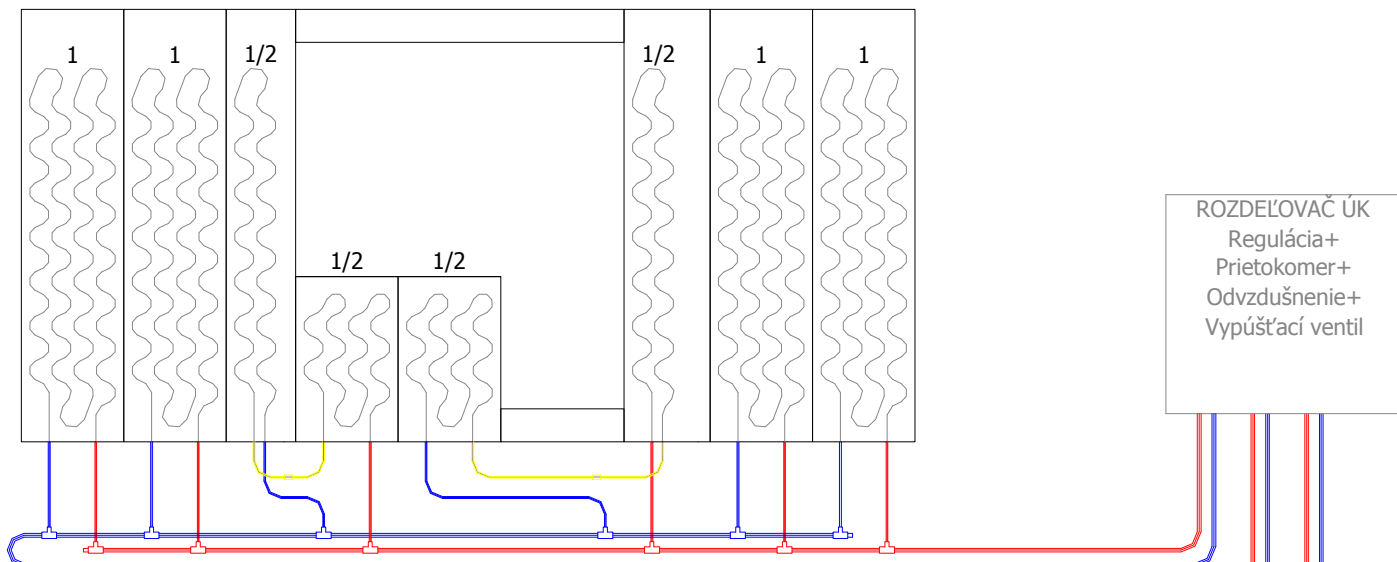
STENA "A" S BALKONOVOU ZOSTAVOU
